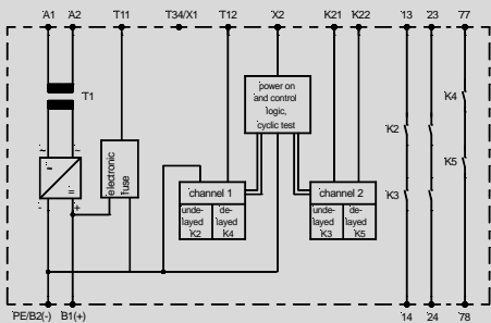
B1(+), PE/B2(-) : 24V DC-Anschluss oder A1, A2 : AC-Anschluss
